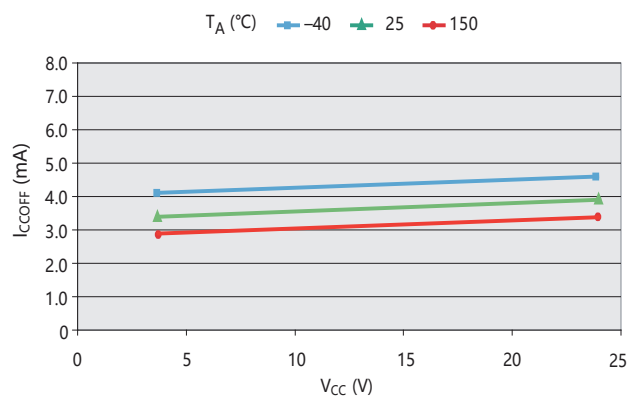
功耗电流(输出截止) VS 工作电压
